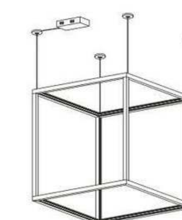
LC-59-E LED:32W L30*W30*H200CM
