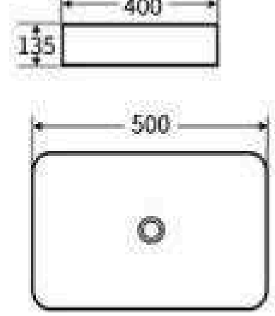
S625 艺术盆 尺寸: 500x400x135mm 台上安装
