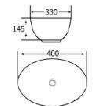
G617 艺术盆 尺寸: 400x330x145mm 台上安装
