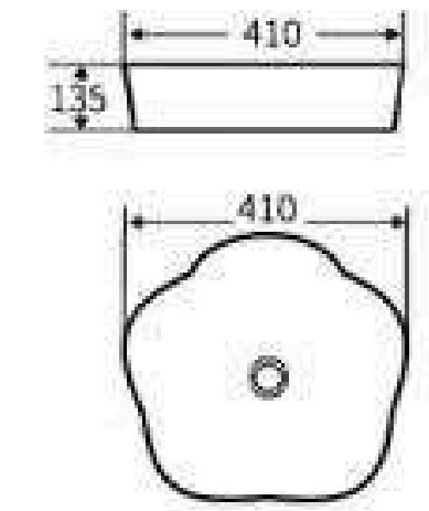
WG634 艺术盆 尺寸: 410x410x135mm 台上安装
