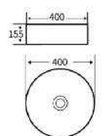
G387 艺术盆 尺寸: 400x400x155mm 台上安装
