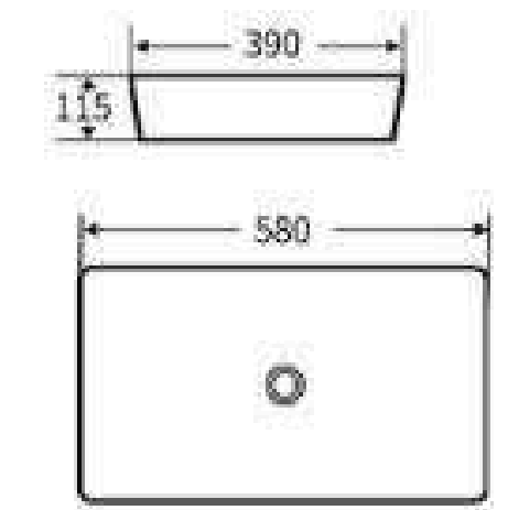
G632 艺术盆 尺寸: 580x390x115mm 台上安装
