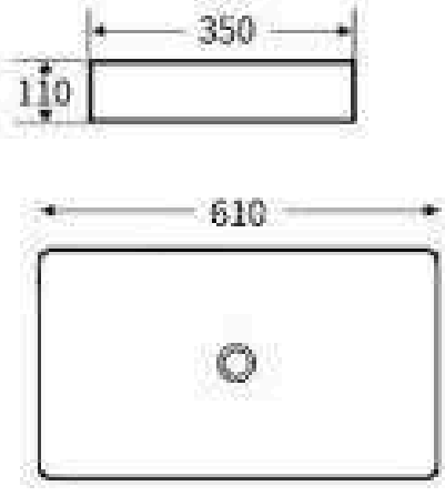
S613 艺术盆 尺寸: 610x350x110mm 台上安装
