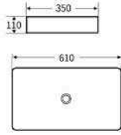
G611 艺术盆 尺寸: 610x350x110mm 台上安装
