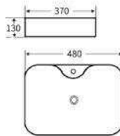
G383 艺术盆 尺寸: 480x370x130mm 台上安装
