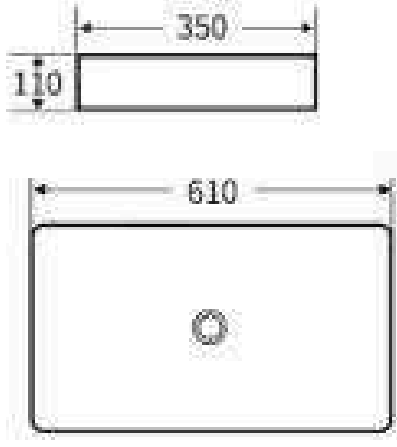
G612 艺术盆 尺寸: 610x350x110mm 台上安装
