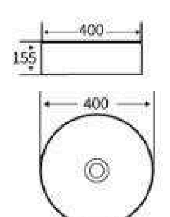
G391 艺术盆 尺寸: 400x400x155mm 台上安装
