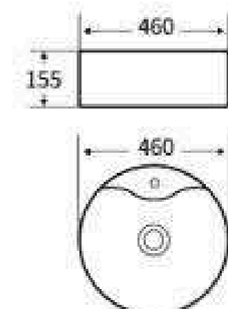
G382 艺术盆 尺寸: 460x460x155mm 台上安装
