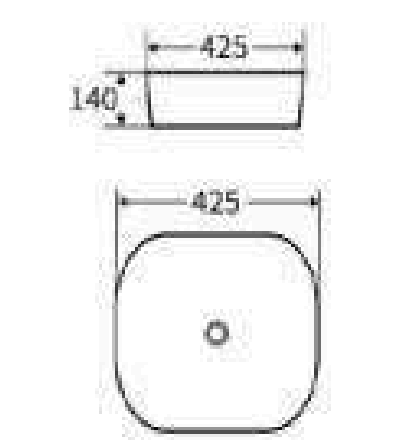
G618 艺术盆 尺寸: 425x425x140mm 台上安装
