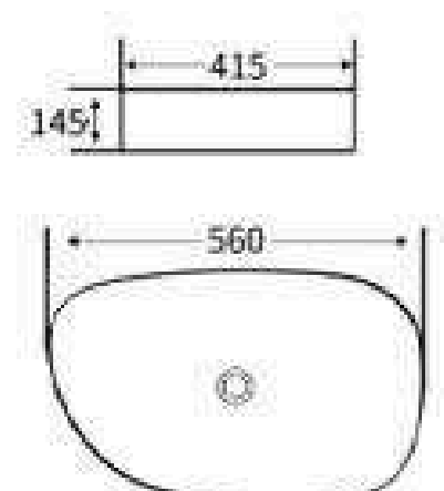
S620 艺术盆 尺寸: 560x415x145mm 台上安装
