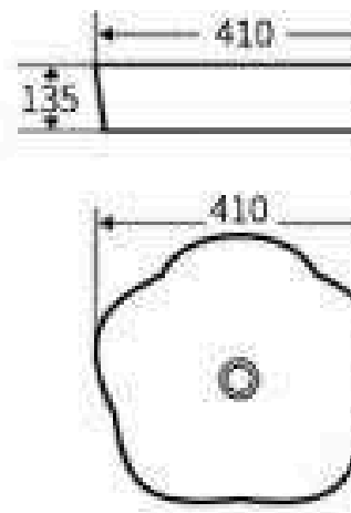
G633 艺术盆 尺寸: 410x410x135mm 台上安装
