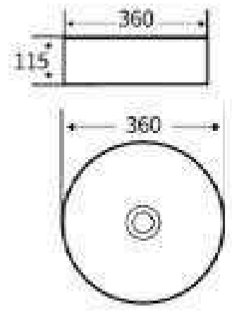
G623 艺术盆 尺寸: 360x360x115mm 台上安装
