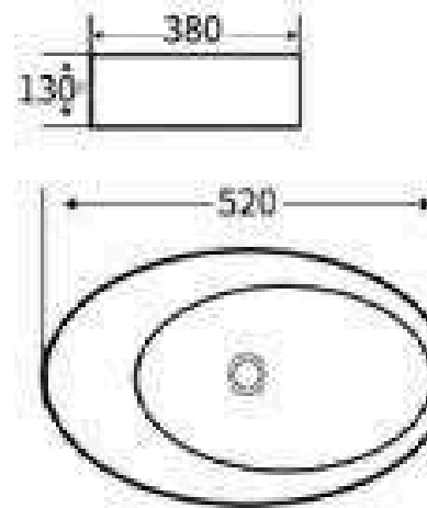
S628 艺术盆 尺寸: 520x380x130mm 台上安装
