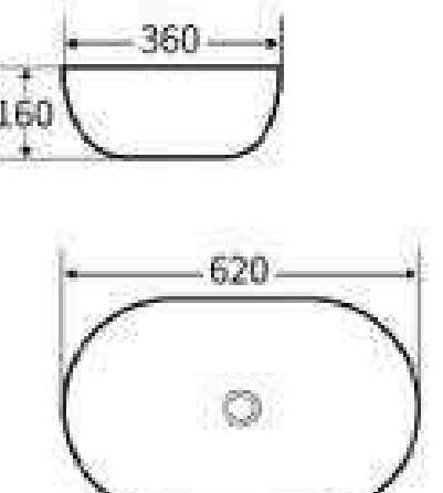
G614 艺术盆 尺寸: 620x360x160mm 台上安装
