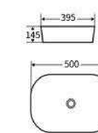
G388 艺术盆 尺寸: 500x395x145mm 台上安装
