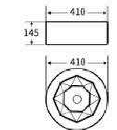
WG616 艺术盆 尺寸: 410x410x145mm 台上安装
