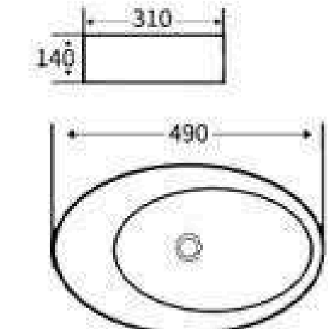
G629 艺术盆 尺寸: 490x310x140mm 台上安装
