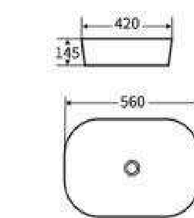
G389 艺术盆 尺寸: 560x420x145mm 台上安装
