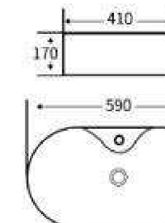
G392 艺术盆 尺寸: 590x410x170mm 台上安装
