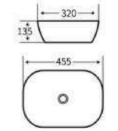
S619 艺术盆 尺寸: 455x320x135mm 台上安装
