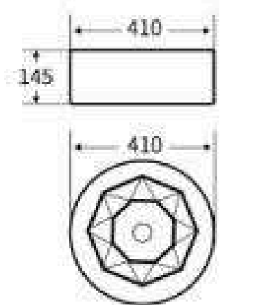
G615 艺术盆 尺寸: 410x410x145mm 台上安装
