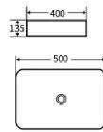
G381 艺术盆 尺寸: 500x400x135mm 台上安装
