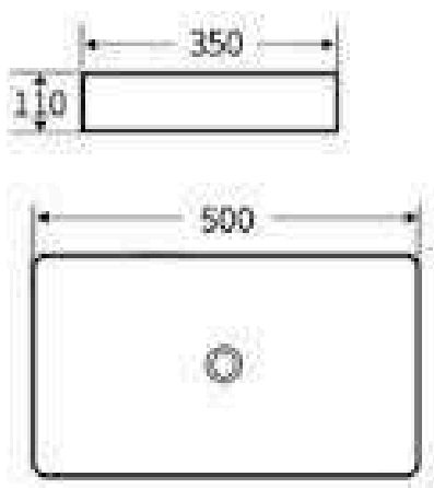
G621 艺术盆 尺寸: 500x350x110mm 台上安装
