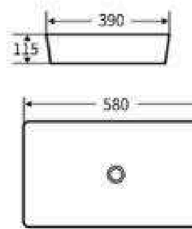
S631 艺术盆 尺寸: 580x390x115mm 台上安装
