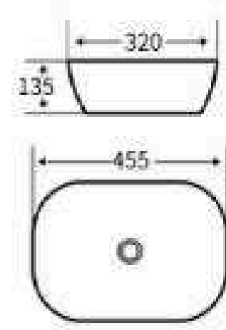
S627 艺术盆 尺寸: 455x320x135mm 台上安装
