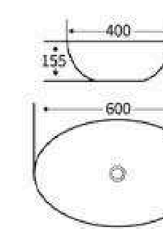
G385 艺术盆 尺寸: 600x400x155mm 台上安装
