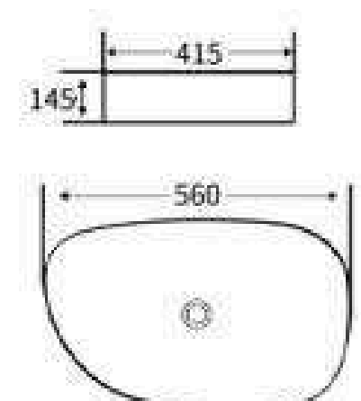
S620 艺术盆 尺寸: 560x415x145mm 台上安装
