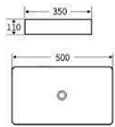
G621 艺术盆 尺寸: 500x350x110mm 台上安装
