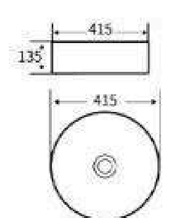
G622 艺术盆 尺寸: 415x415x135mm 台上安装
